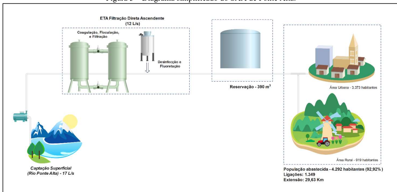
Figura 5 – Diagrama simplificado do SAA de Ponte Alta.
