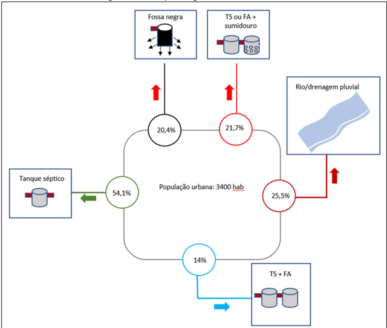
Figura 8 - Distribuição do esgoto na área urbana de Ponte Alta.
