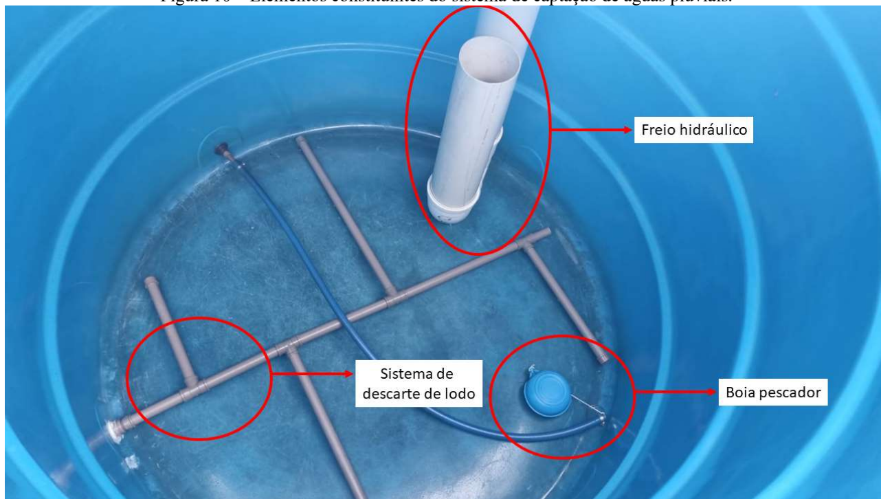
Figura 10 – Elementos constituintes do sistema de captação de águas pluviais.
