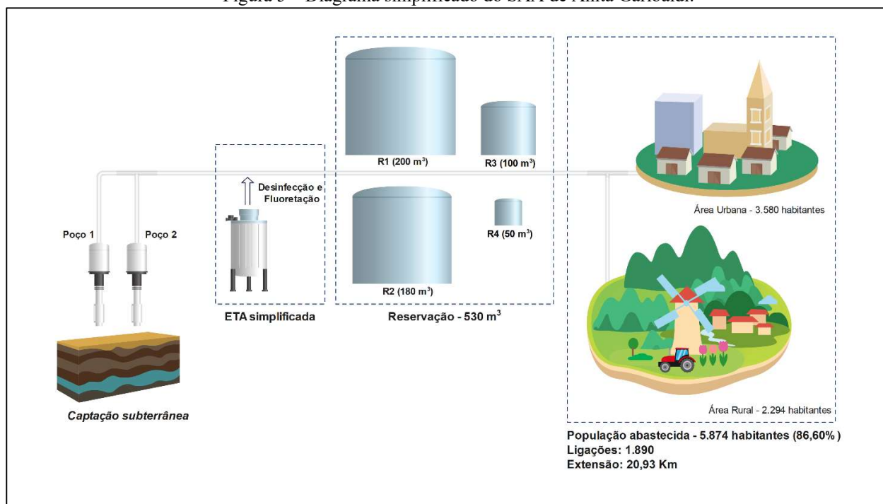
Figura 5 – Diagrama simplificado do SAA de Anita Garibaldi.
